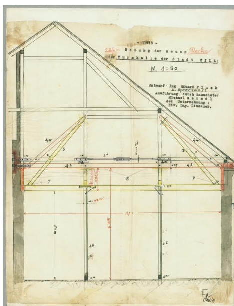
Slika 14: Načrt telovadnice z arhitektovim podpisom. Vir: Deželni arhiv Gradec
