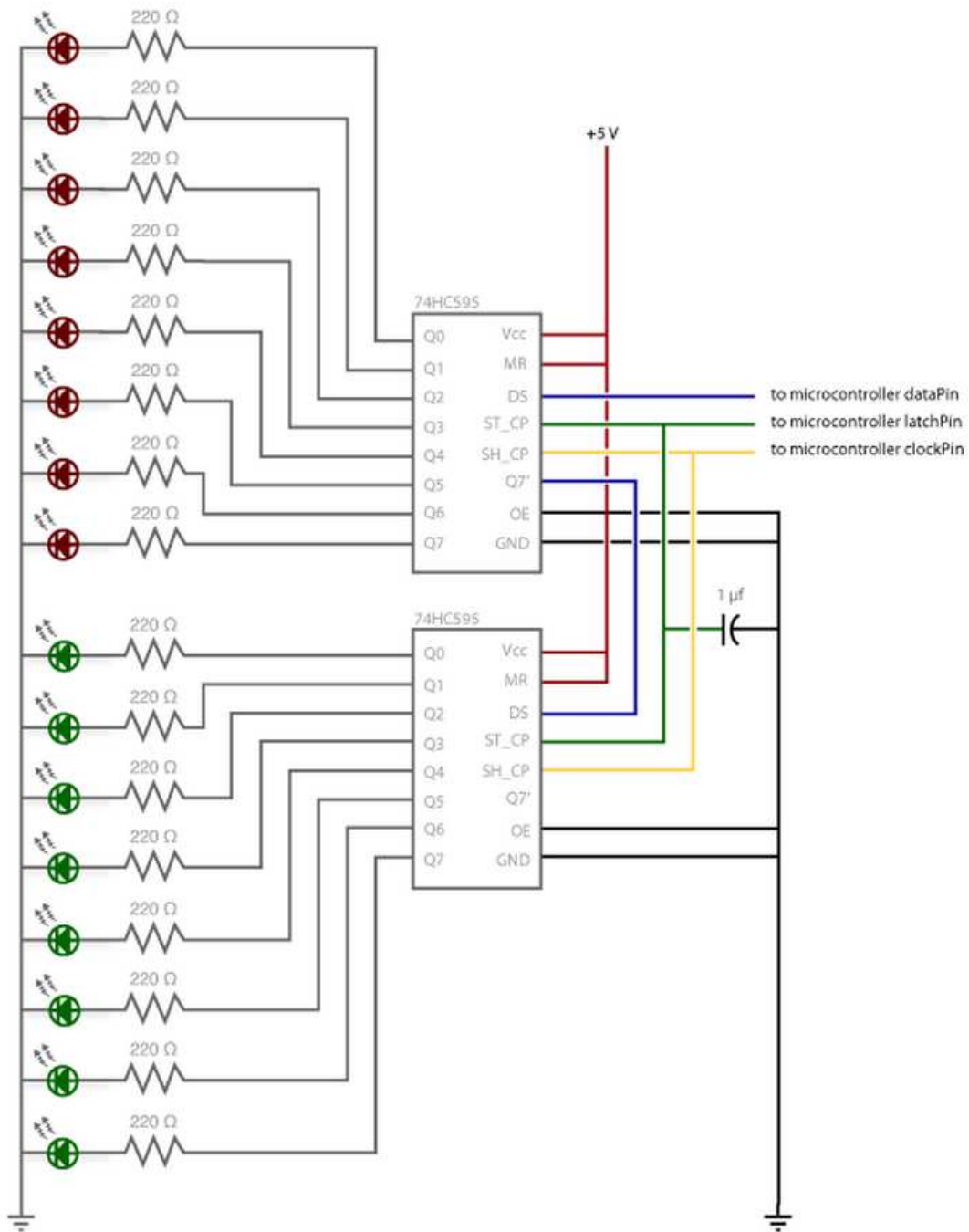
Slika 9: Primer vezave čipov 74HC595
