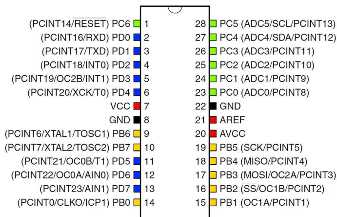
Slika 7: Razvrstitev pinov na mikročipu
