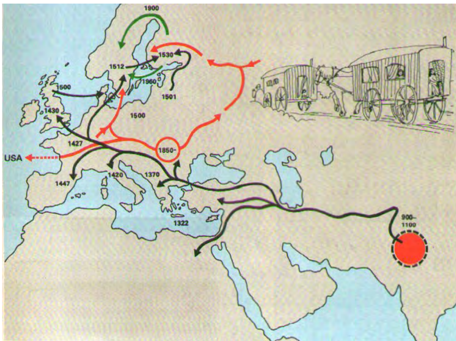
Slika 2: Priseljevanje Romov
