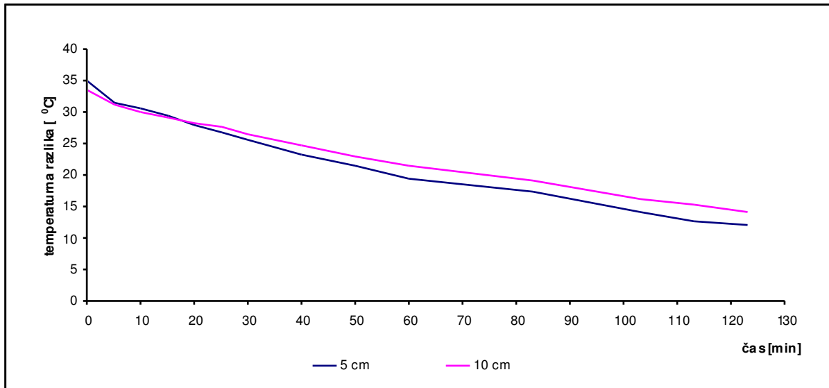
Graf št. 1: Temperaturne razlike v časovnih presledkih – različni debelini izolacije
