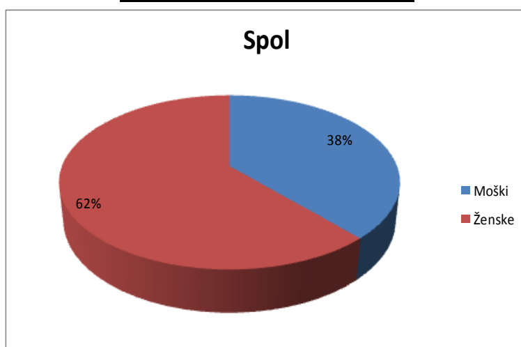
Slika 5: Graf 1
