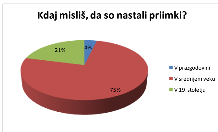
Slika 12: Graf 6
