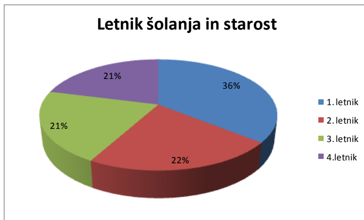
Slika 6: Graf 2
